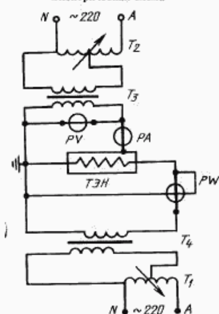
Электрическая схема
