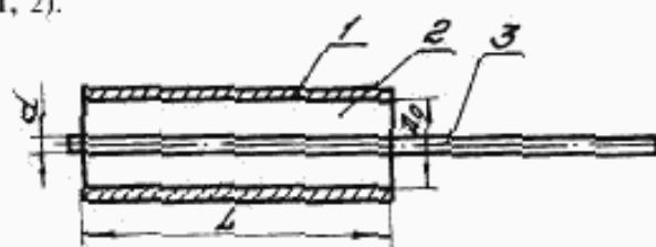
1 — оболочка; 2 — уплотненный порошок; 3 — стержень
